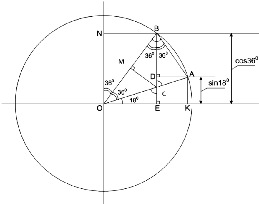
Рис. 1. Геометрическое представление тождества (3)
